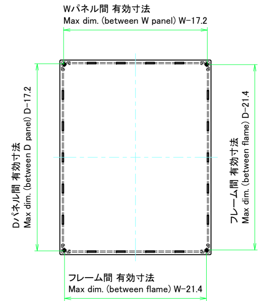
下カバー / Bottom cover
