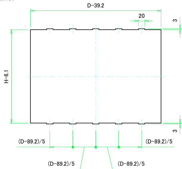
Dパネル1表面 / D Panel 1 Frontside
